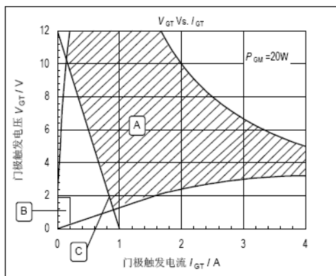
图9. 门极触发特性曲线 Fig9. Gate parameter curve
