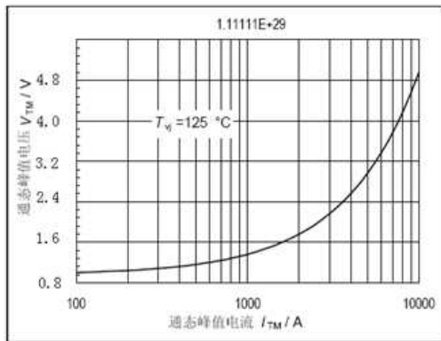
图1. 通态伏安特性曲线
