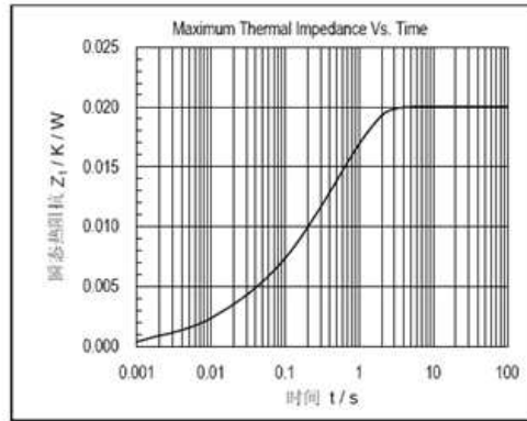
图2. 瞬态热阻抗曲线
