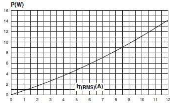
图3 通态特性
