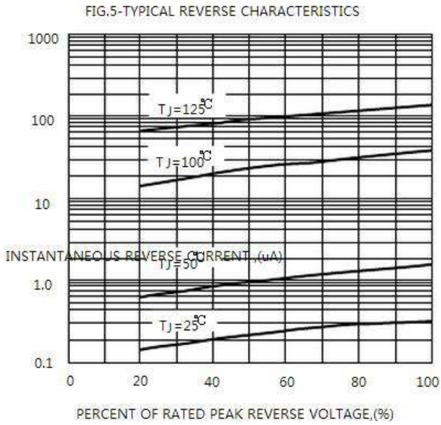
图5. 典型反向特性曲线
